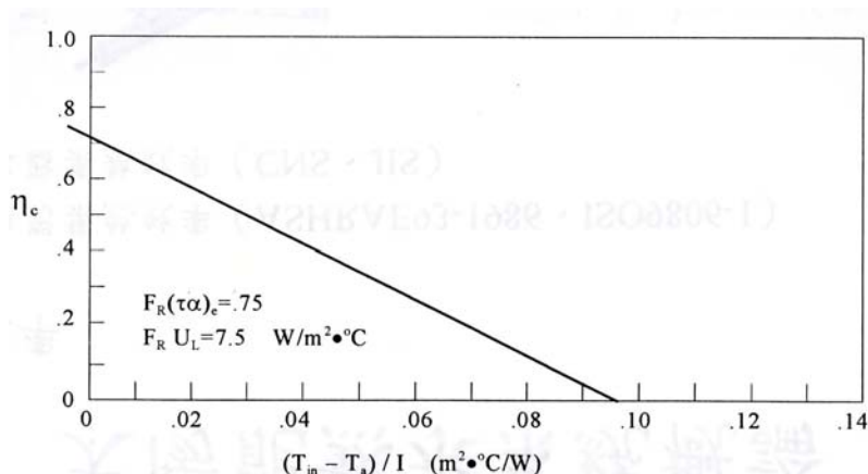
圖 4-4-10 熱傳效率性能效率曲線圖
