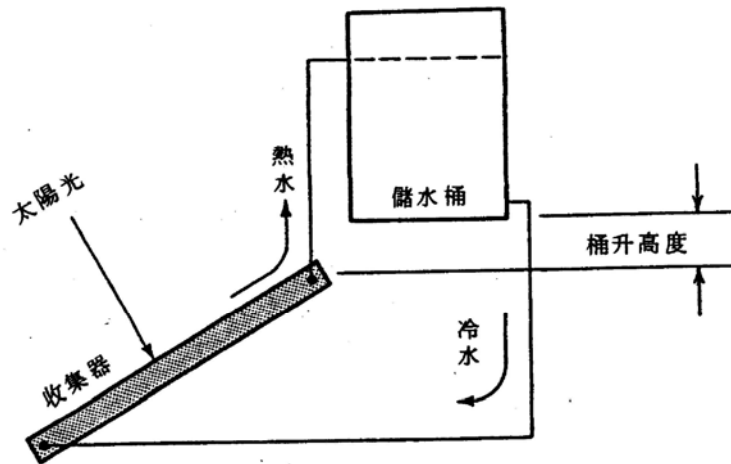
圖 4-4-6 典型的自然循環式太陽能熱水系統【12】
