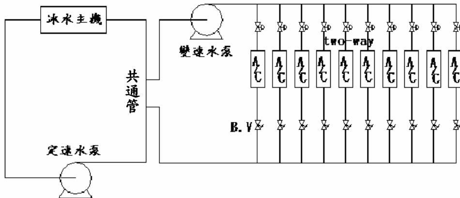
圖 4-5-12 P-S 系統圖【9】
