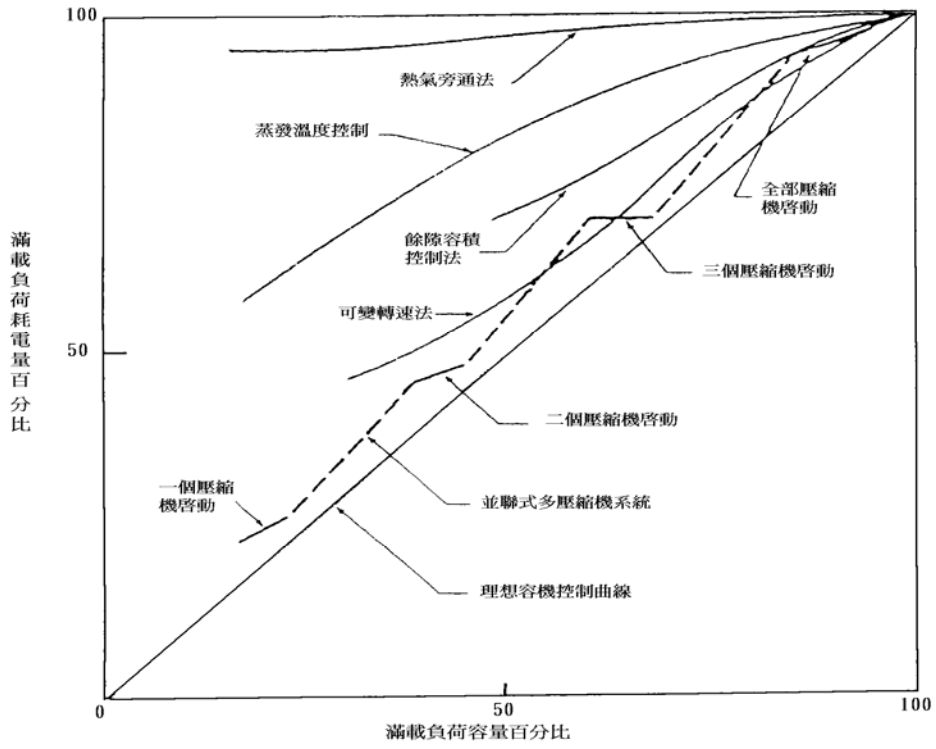
圖 4-5-5 壓縮機的容量控制圖【11】
