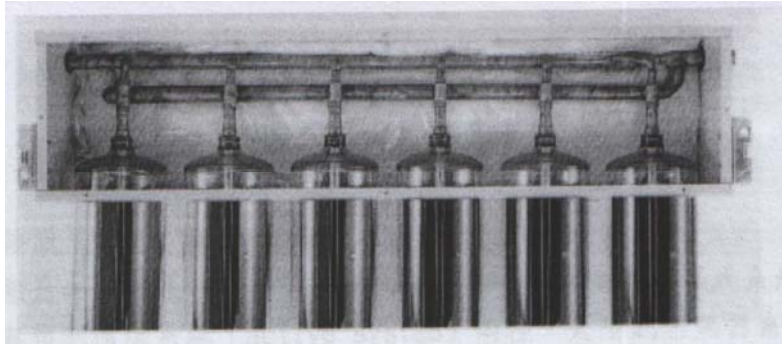
圖 4-4-5 銅鰭片銅管式真空管集熱器【5】
